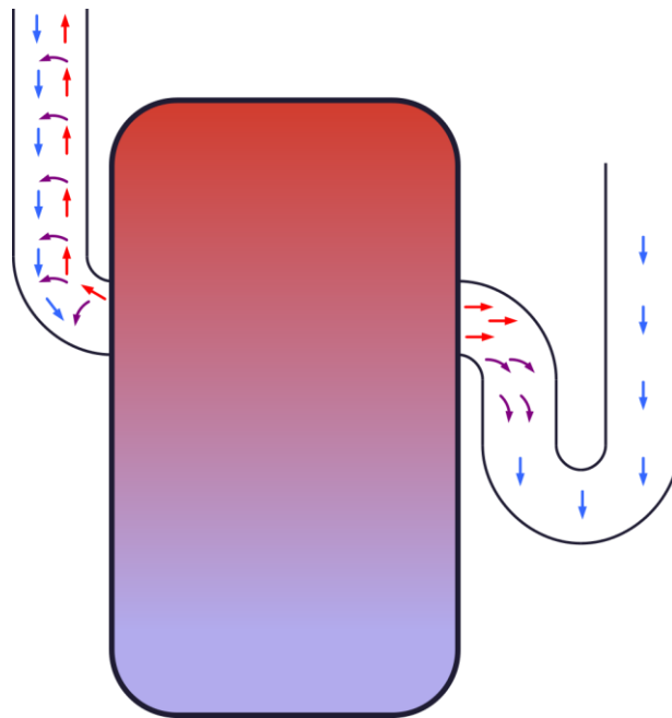
Abbildung 21: Speicherauskuhlung durch Gegenstromzirkulation (links) und Gegenmaßnahme Thermosiphon (rechts)
